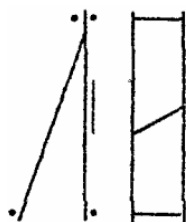
Рис. 2. Полуанкерная опора
